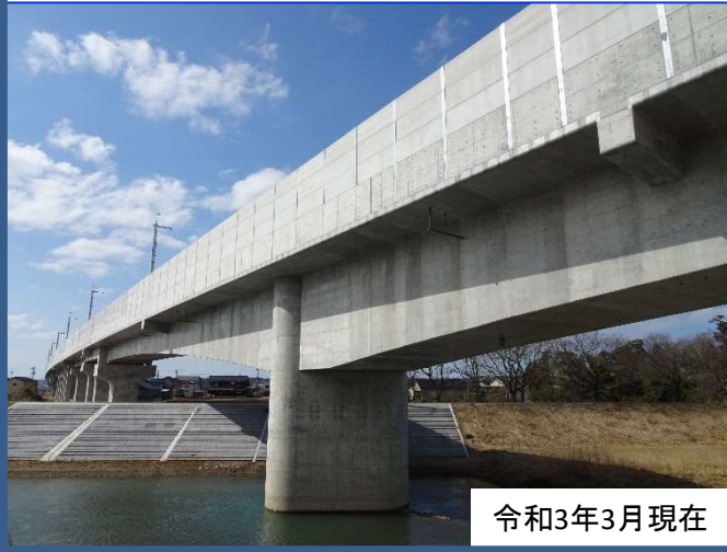
動橋川橋りょう【加賀市】
