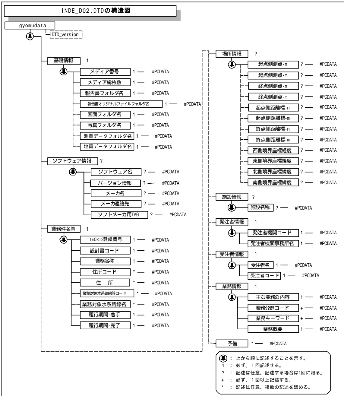
図 1 「INDE_D02.DTD」の構造図
