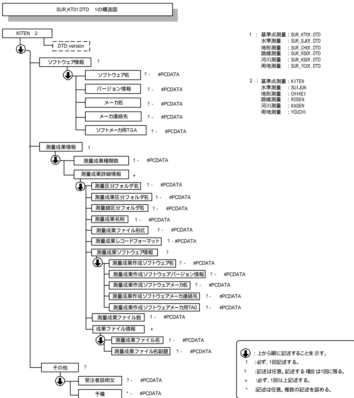
図 3 「SUR_KT01.DTD」の構造図
