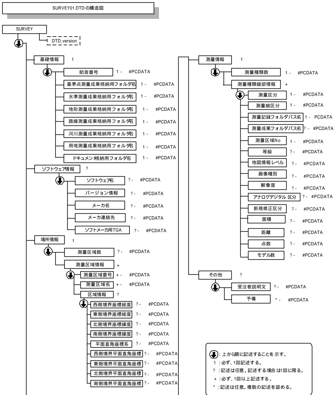
図 2 「SURVEY01.DTD」の構造図
